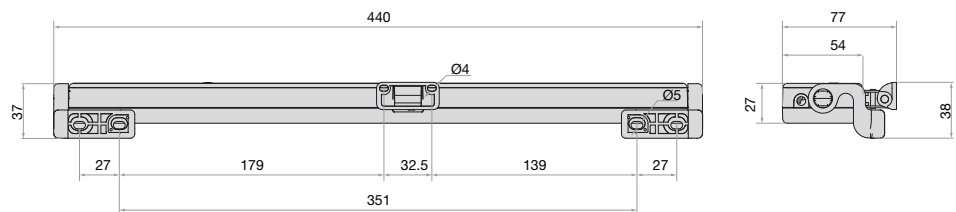
Dimenzije preklopni prozor
