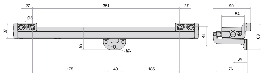
Dimenzije nagibni prozor
